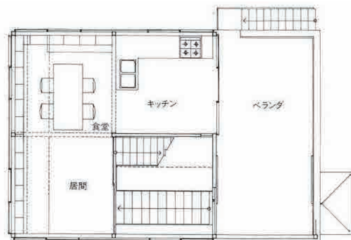
2階平面
