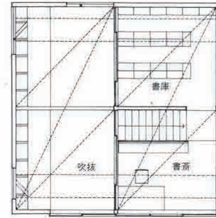
3階平面
